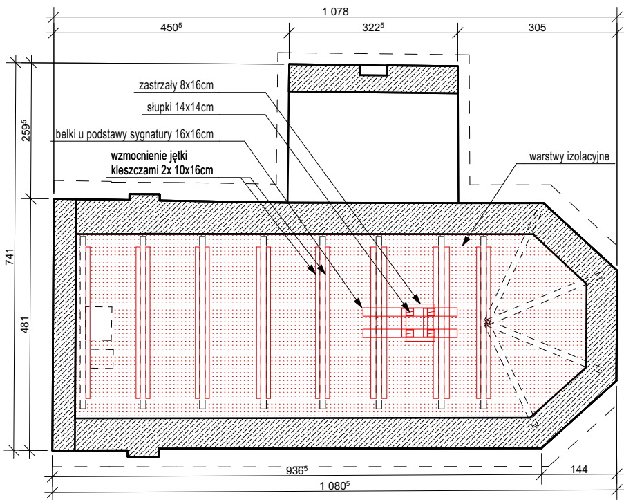
RZUT PODDASZA NIEUŻYTKOWEGO
