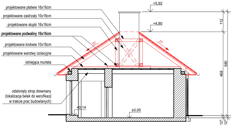
PRZĘKRÓJ POPRZECZNY
