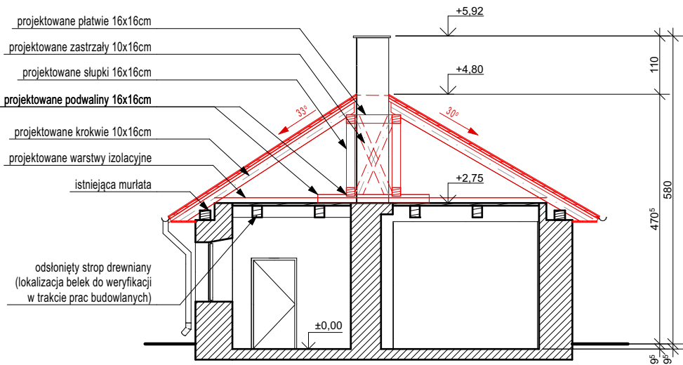
PRZĘKRÓJ PODŁUŻNY
