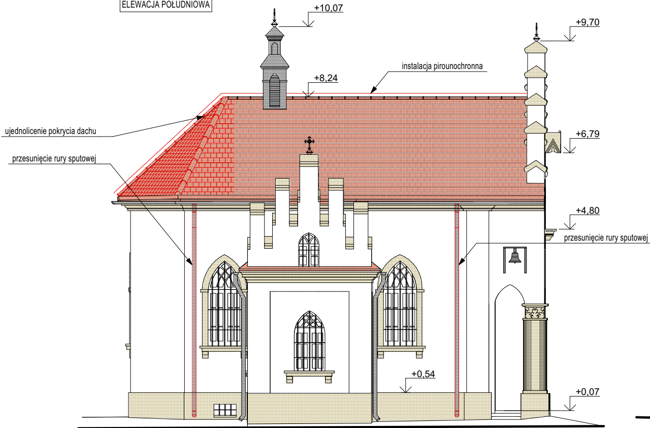
ELEWACJA POŁUDNIOWA
