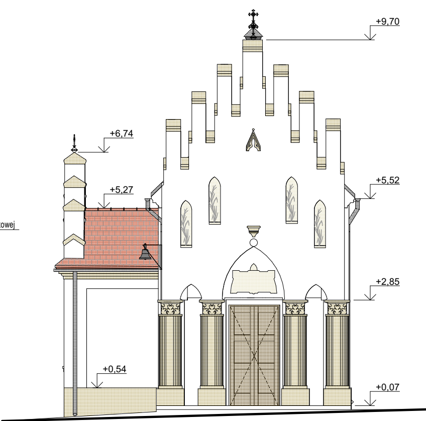
ELEWACJA WSCHODNIA
