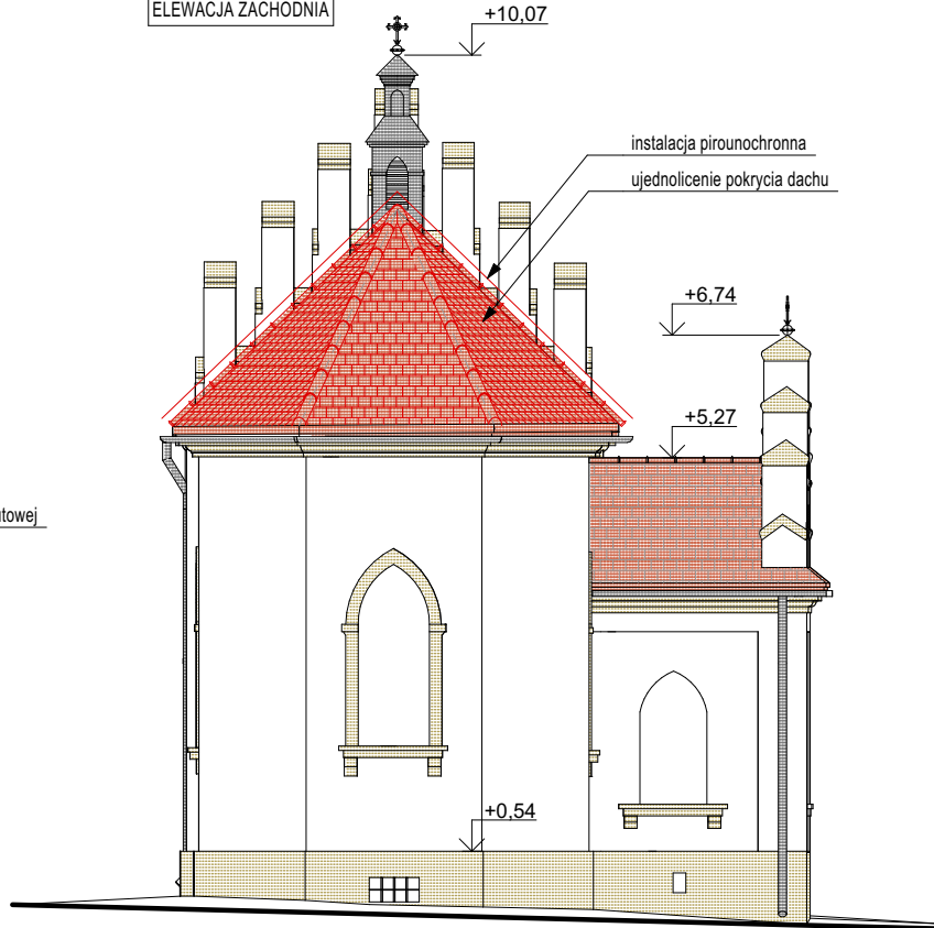
ELEWACJA ZACHODNIA
