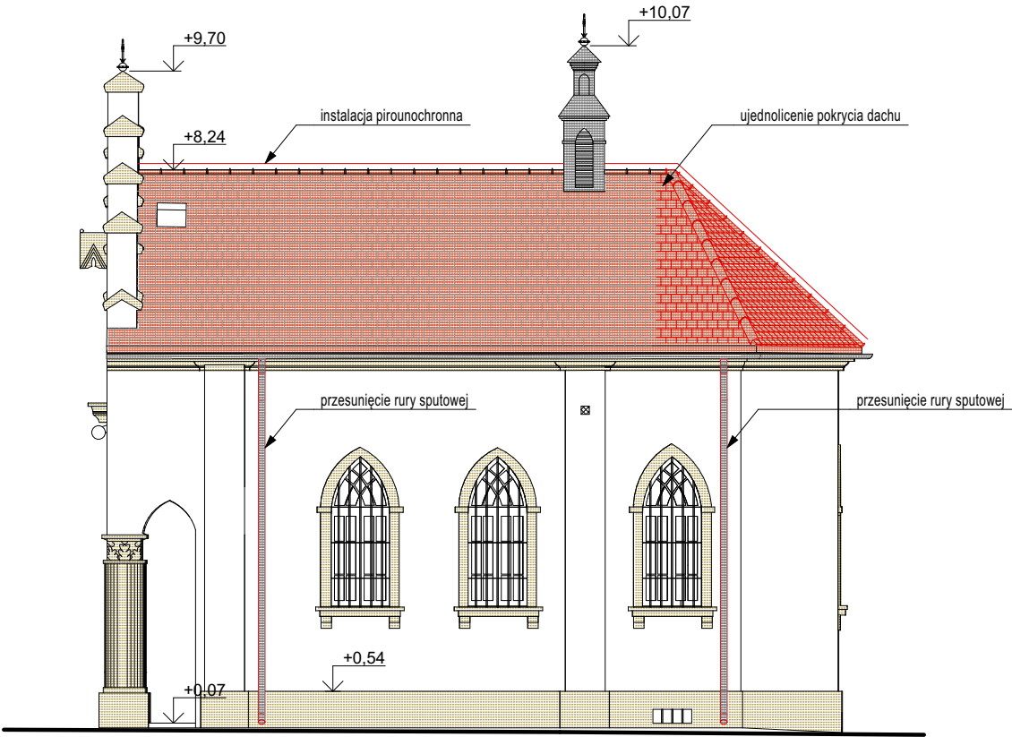
ELEWACJA PÓŁNOCNA
